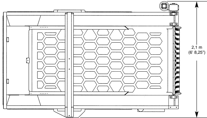
Enfriador Compacto Modelo LCC (Vista Superior)
