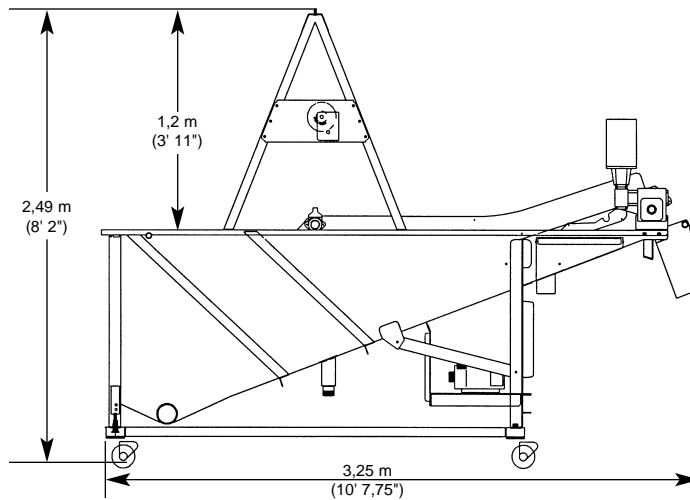
Enfriador Compacto Modelo LCC (Vista Lateral)
