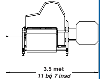
HÌNH CHIẾU CẠNH (hình cửa đang mở)
